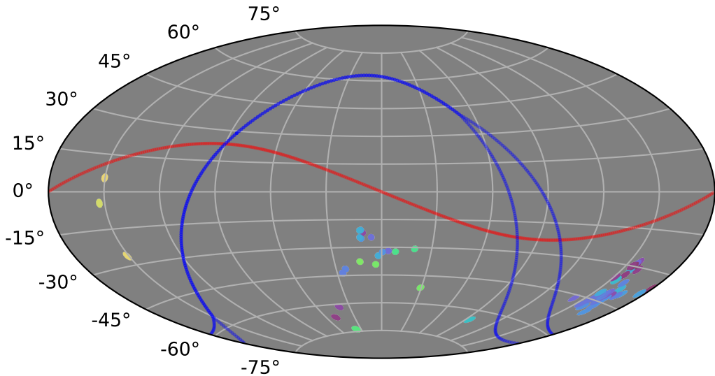
weather_cloudso35v3.4_10yrs gi: LVDwarfs
