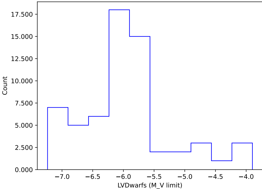
weather_cloudso35v3.4_10yrs gi: LVDwarfs
