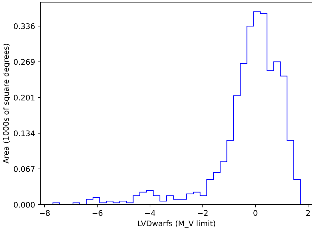
weather_cloudso35v3.4_10yrs gi SCP: LVDwarfs
