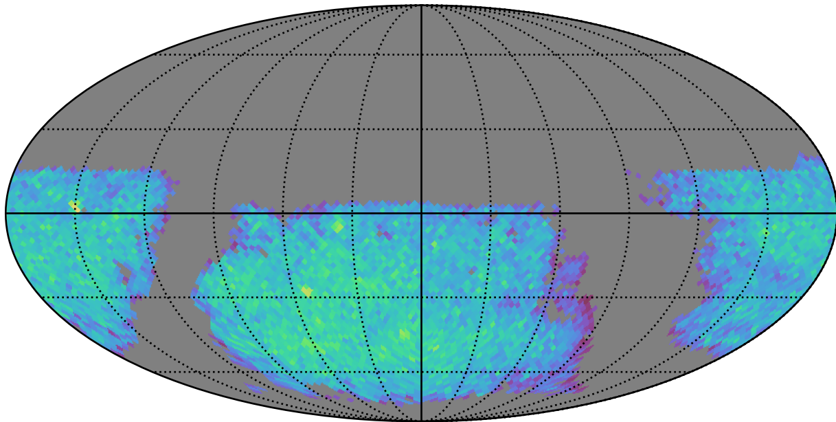
weather_cloudso35v3.4_10yrs gi: LVDwarfs
