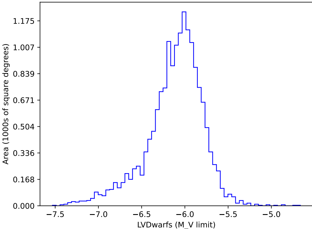
weather_cloudso35v3.4_10yrs gi: LVDwarfs
