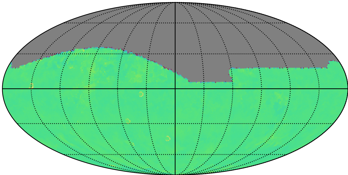
weather_cloudso35v3.4_10yrs z: Kuiper rotTelPos
