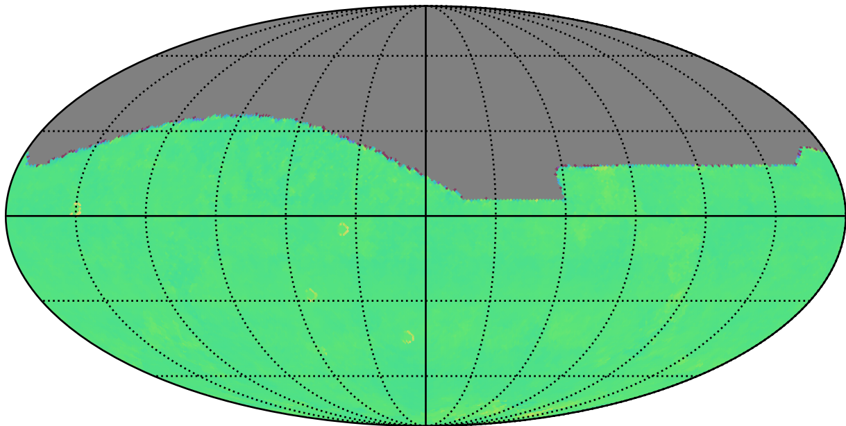
weather_cloudso35v3.4_10yrs r: Kuiper rotTelPos
