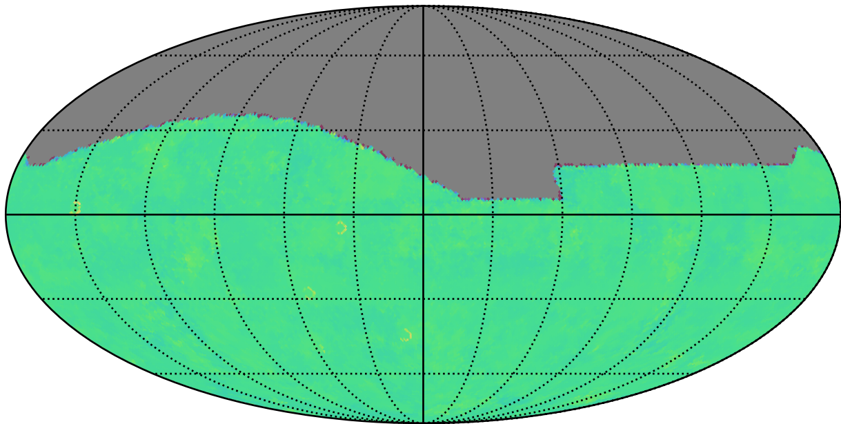
weather_cloudso35v3.4_10yrs g: Kuiper rotTelPos
