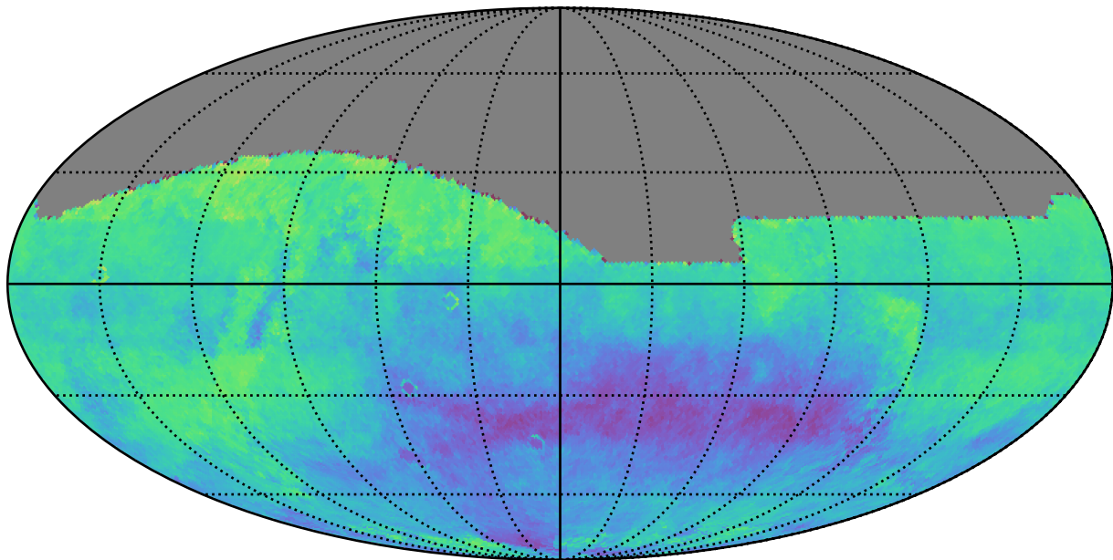
weather_cloudso35v3.4_10yrs z: Kuiper rotSkyPos
