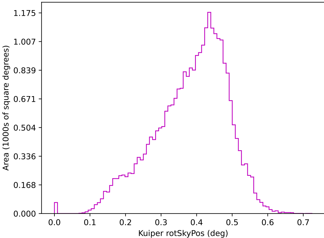
weather_cloudso35v3.4_10yrs z: Kuiper rotSkyPos
