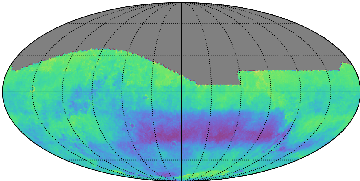
weather_cloudso35v3.4_10yrs r: Kuiper rotSkyPos
