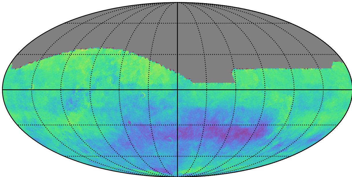
weather_cloudso35v3.4_10yrs i: Kuiper rotSkyPos
