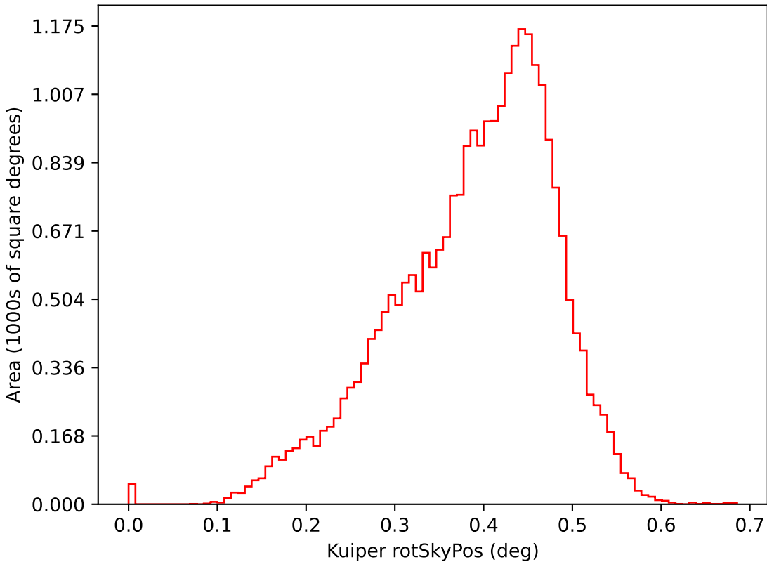
weather_cloudso35v3.4_10yrs i: Kuiper rotSkyPos
