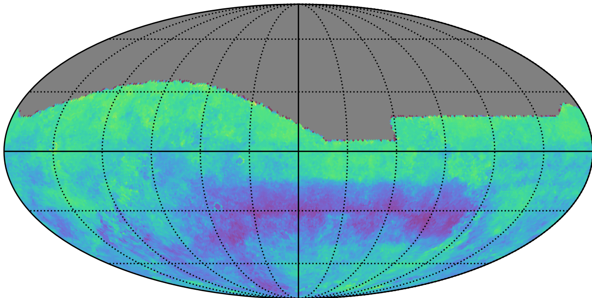
weather_cloudso35v3.4_10yrs g: Kuiper rotSkyPos
