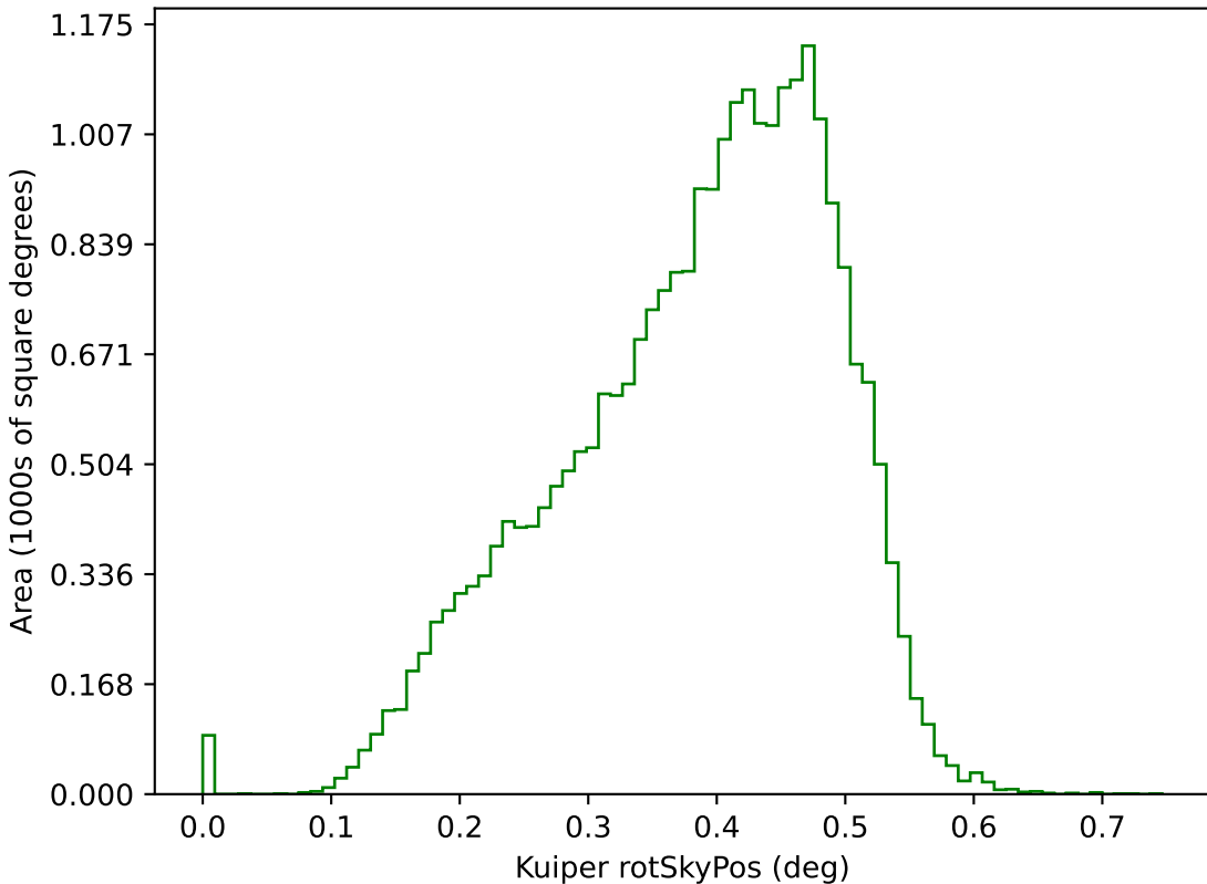
weather_cloudso35v3.4_10yrs g: Kuiper rotSkyPos
