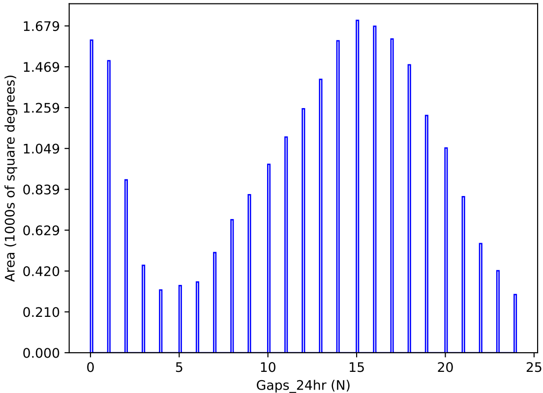
weather_cloudso35v3.4_10yrs y band: Gaps_24hr
