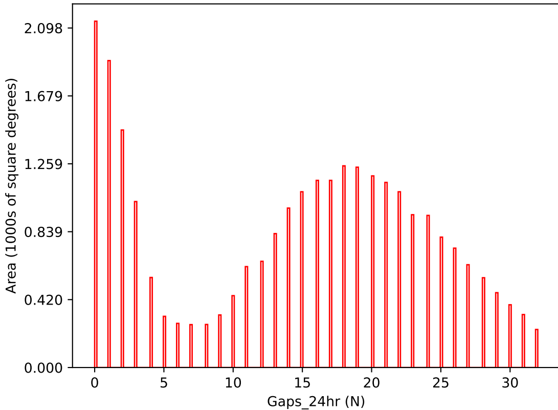
weather_cloudso35v3.4_10yrs i band: Gaps_24hr
