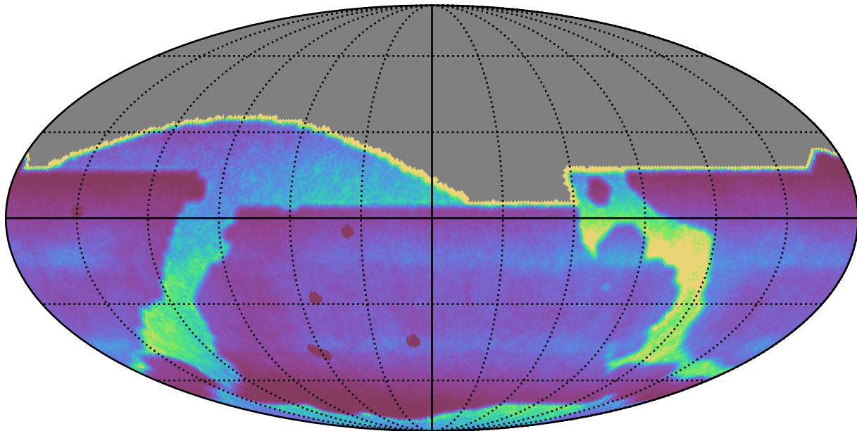
weather_cloudso35v3.4_10yrs : DCRprecision
