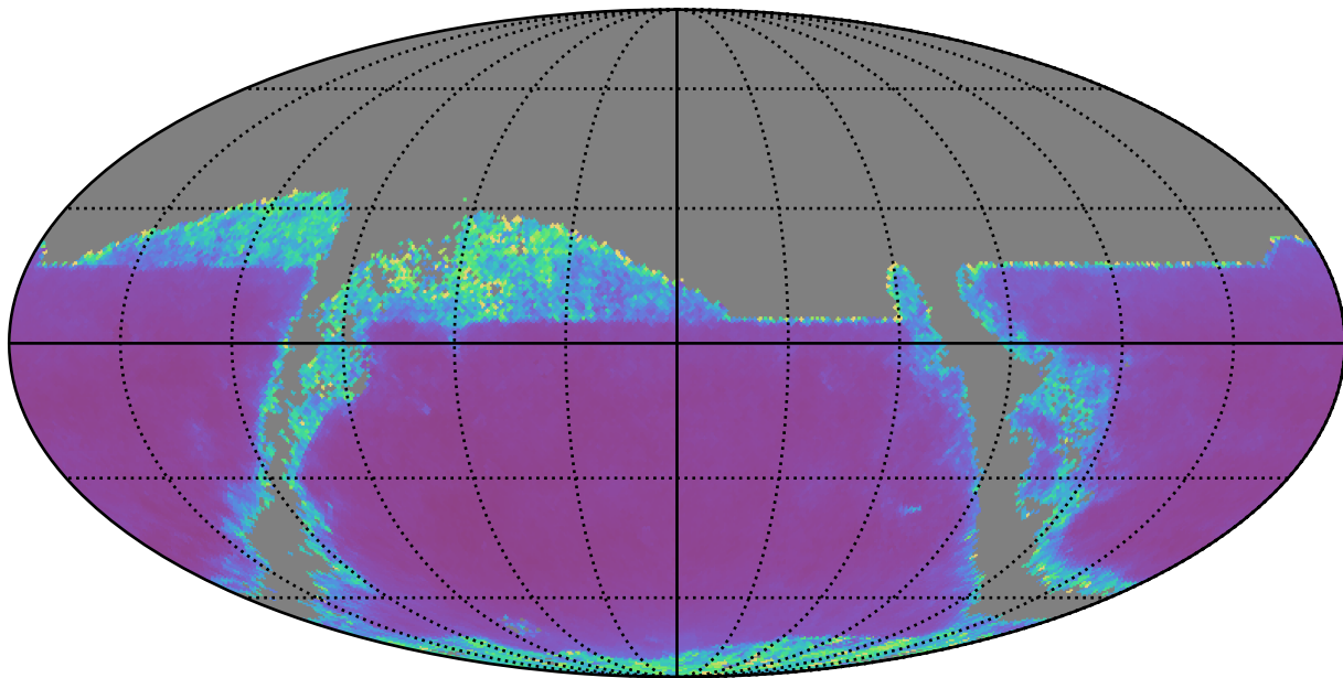
weather_cloudso35v3.4_10yrs z band: AGN SF_uncert
