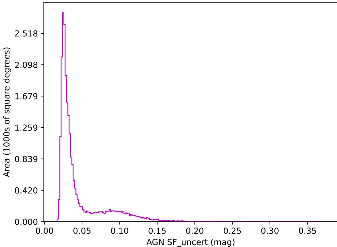
weather_cloudso35v3.4_10yrs z band: AGN SF_uncert
