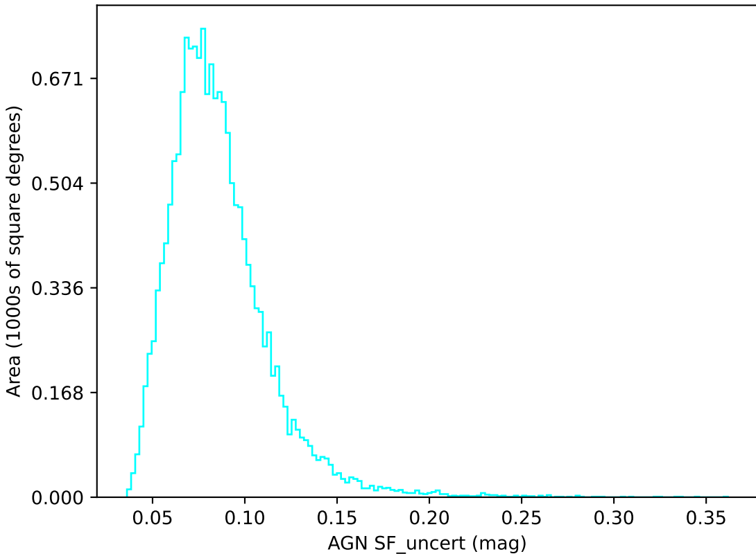
weather_cloudso35v3.4_10yrs u band: AGN SF_uncert
