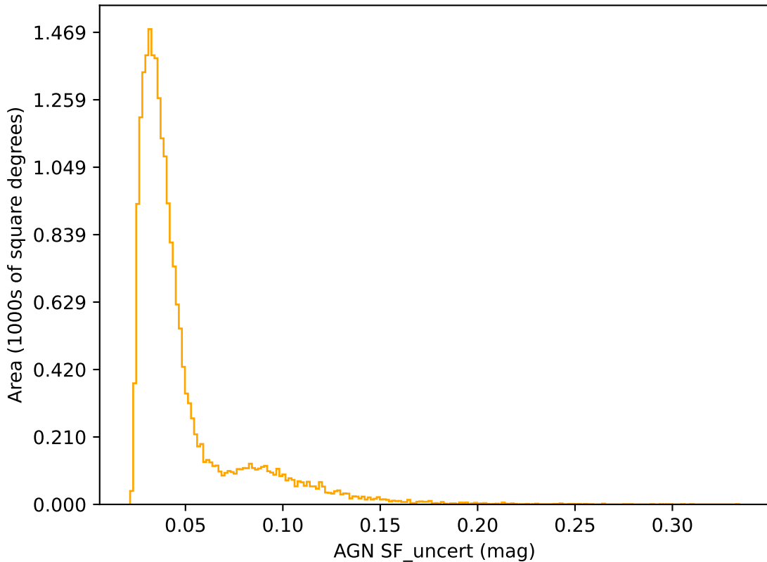
weather_cloudso35v3.4_10yrs r band: AGN SF_uncert
