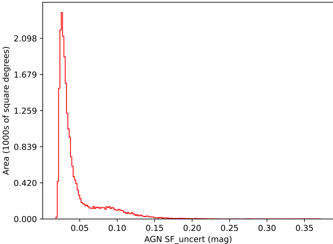
weather_cloudso35v3.4_10yrs i band: AGN SF_uncert
