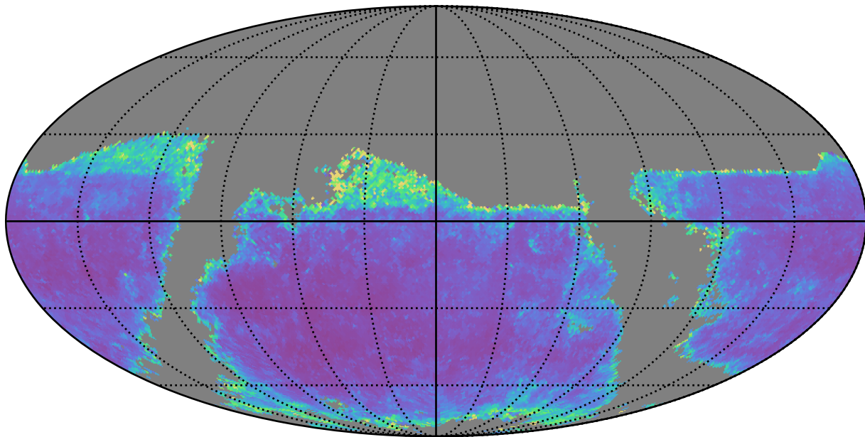
weather_cloudso35v3.4_10yrs g band: AGN SF_uncert
