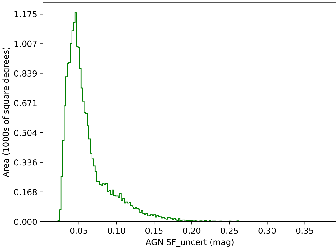
weather_cloudso35v3.4_10yrs g band: AGN SF_uncert
