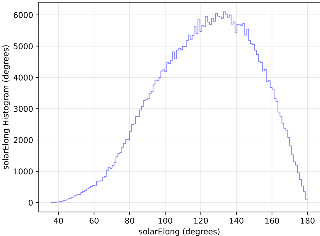
weather_cloudso35v3.4_10yrs WFD y band: solarElong Histogram
