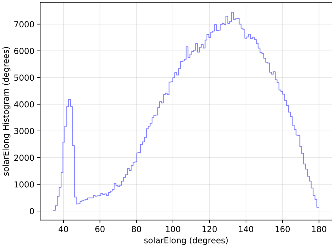
weather_cloudso35v3.4_10yrs All sky i band: solarElong Histogram
