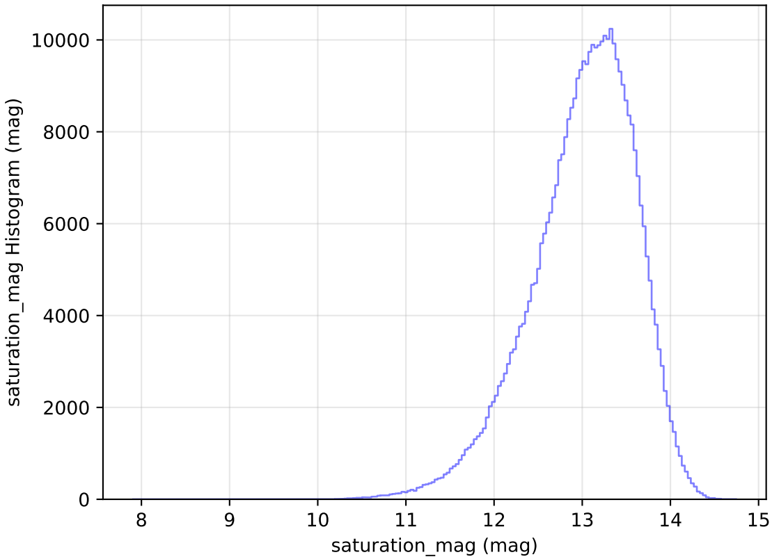
weather_cloudso35v3.4_10yrs WFD y band: saturation_mag Histogram
