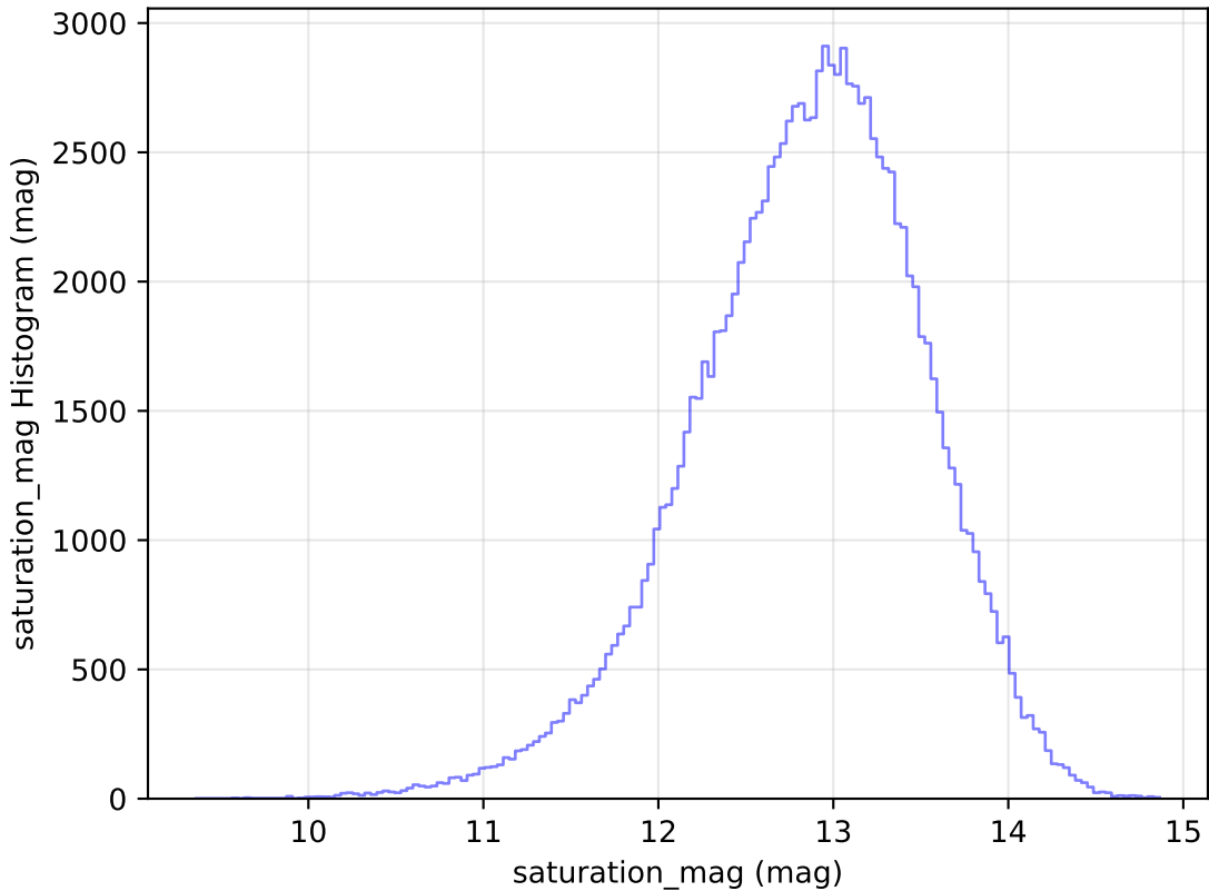
weather_cloudso35v3.4_10yrs WFD u band: saturation_mag Histogram
