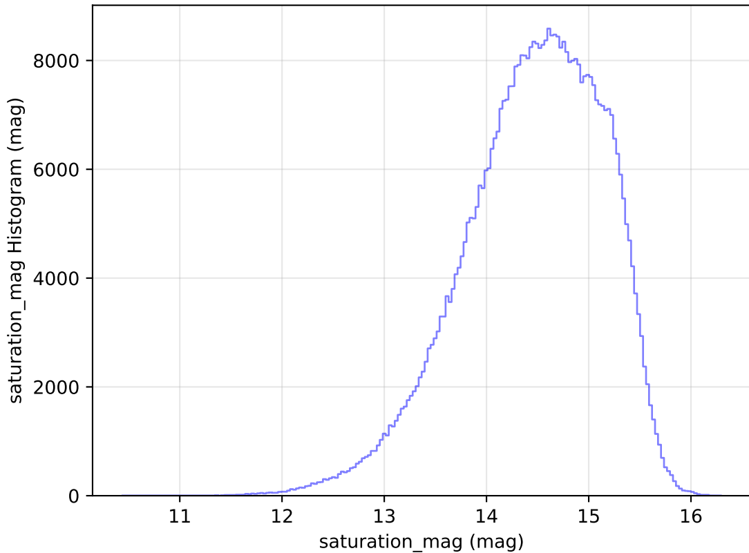
weather_cloudso35v3.4_10yrs WFD r band: saturation_mag Histogram
