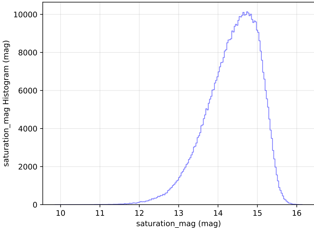
weather_cloudso35v3.4_10yrs WFD i band: saturation_mag Histogram
