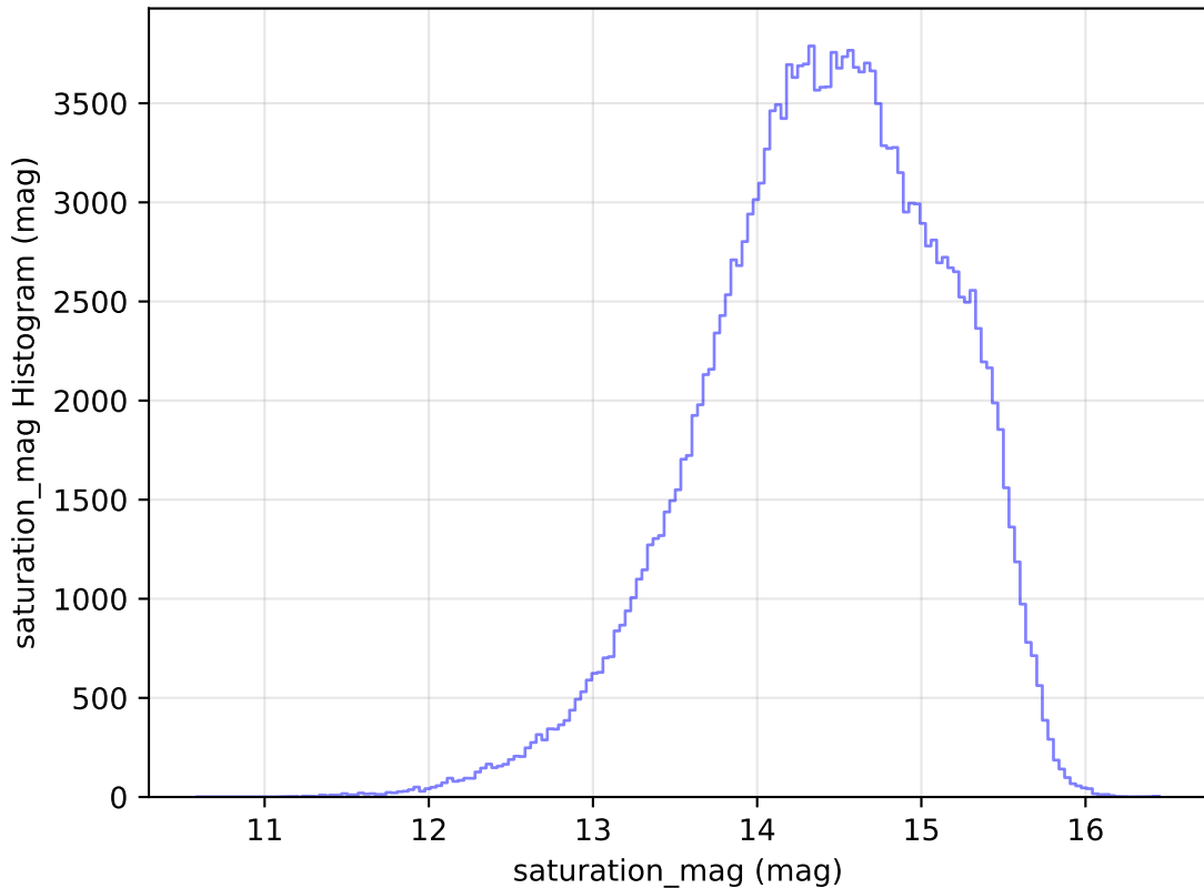
weather_cloudso35v3.4_10yrs WFD g band: saturation_mag Histogram
