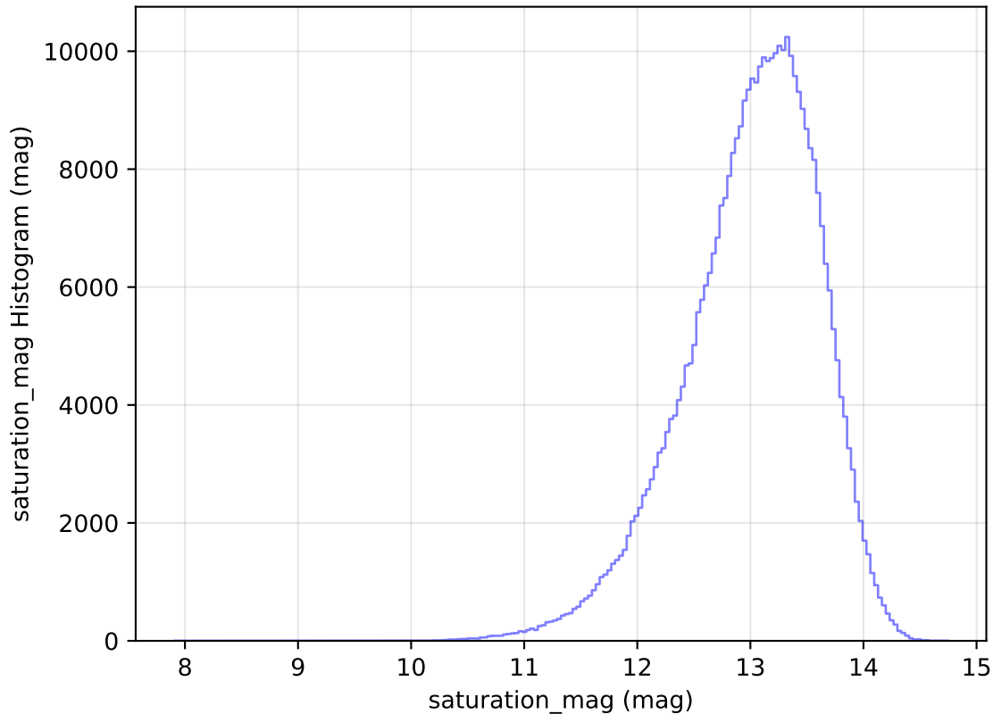
weather_cloudso35v3.4_10yrs All sky y band: saturation_mag Histogram
