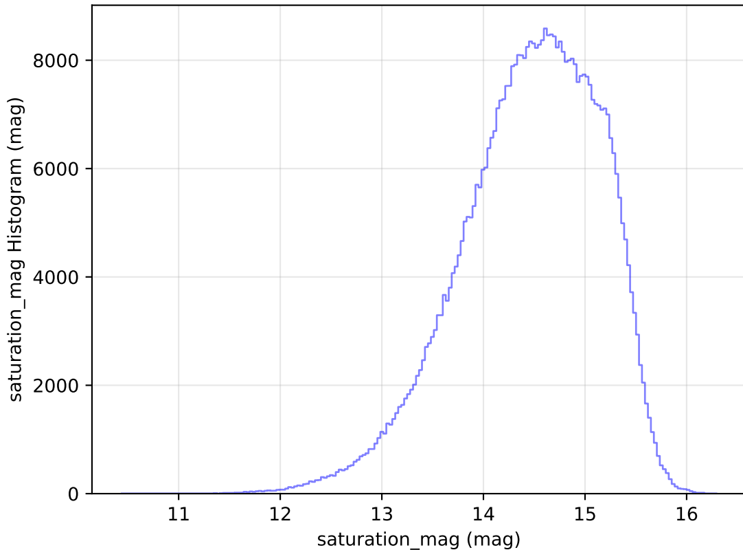
weather_cloudso35v3.4_10yrs All sky r band: saturation_mag Histogram
