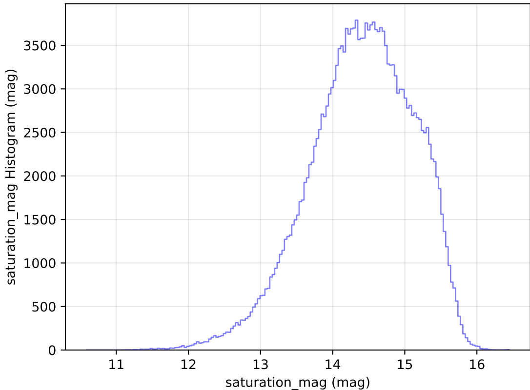
weather_cloudso35v3.4_10yrs All sky g band: saturation_mag Histogram
