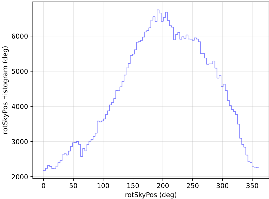
weather_cloudso35v3.4_10yrs WFD z band: rotSkyPos Histogram
