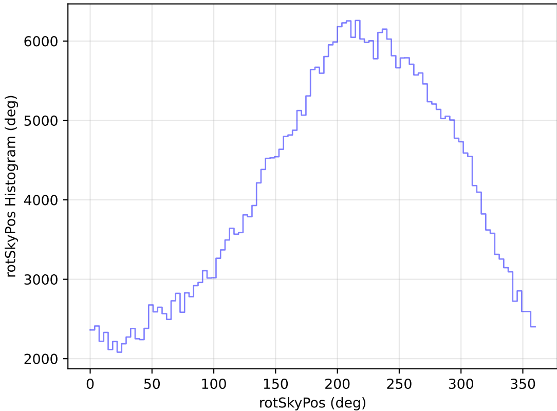
weather_cloudso35v3.4_10yrs WFD y band: rotSkyPos Histogram
