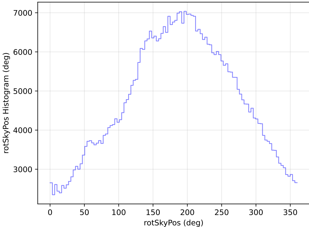
weather_cloudso35v3.4_10yrs WFD r band: rotSkyPos Histogram
