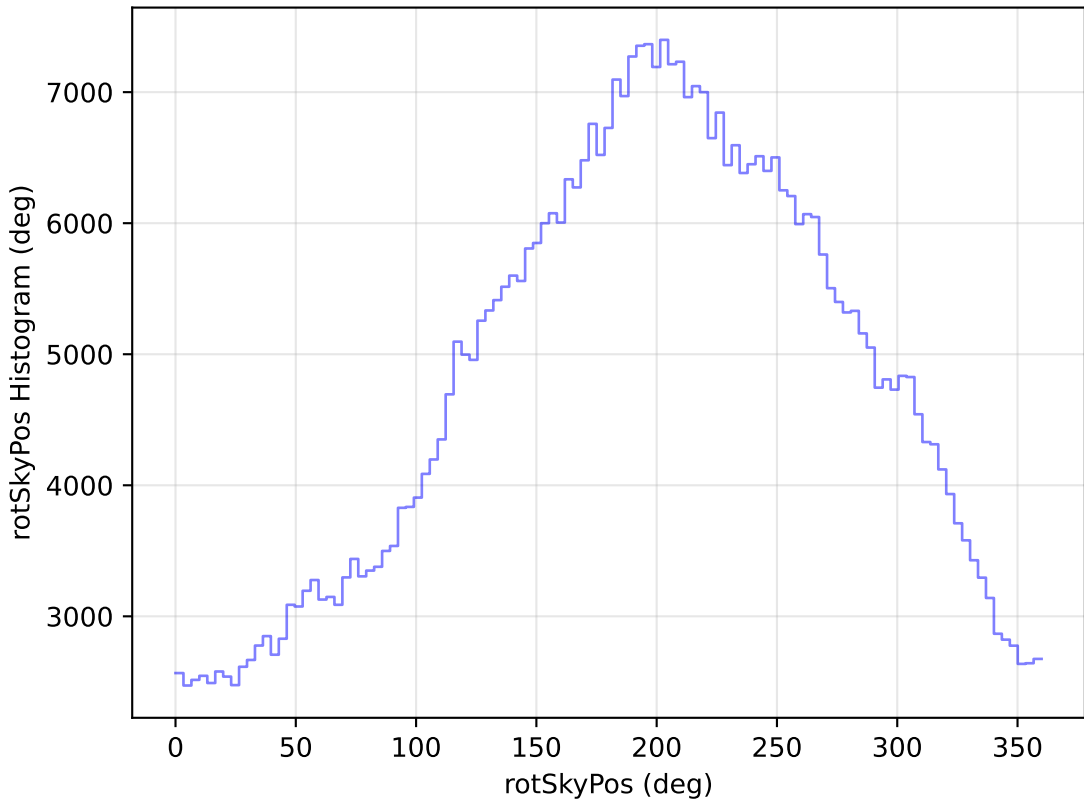
weather_cloudso35v3.4_10yrs WFD i band: rotSkyPos Histogram
