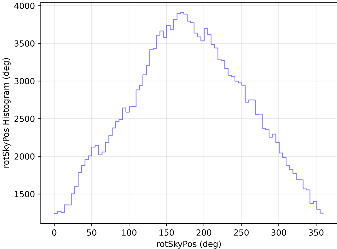
weather_cloudso35v3.4_10yrs WFD g band: rotSkyPos Histogram
