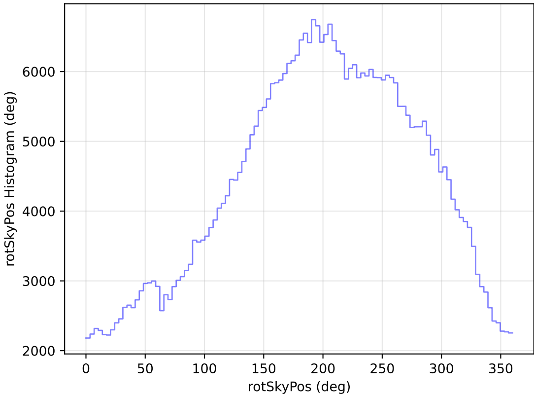
weather_cloudso35v3.4_10yrs All sky z band: rotSkyPos Histogram
