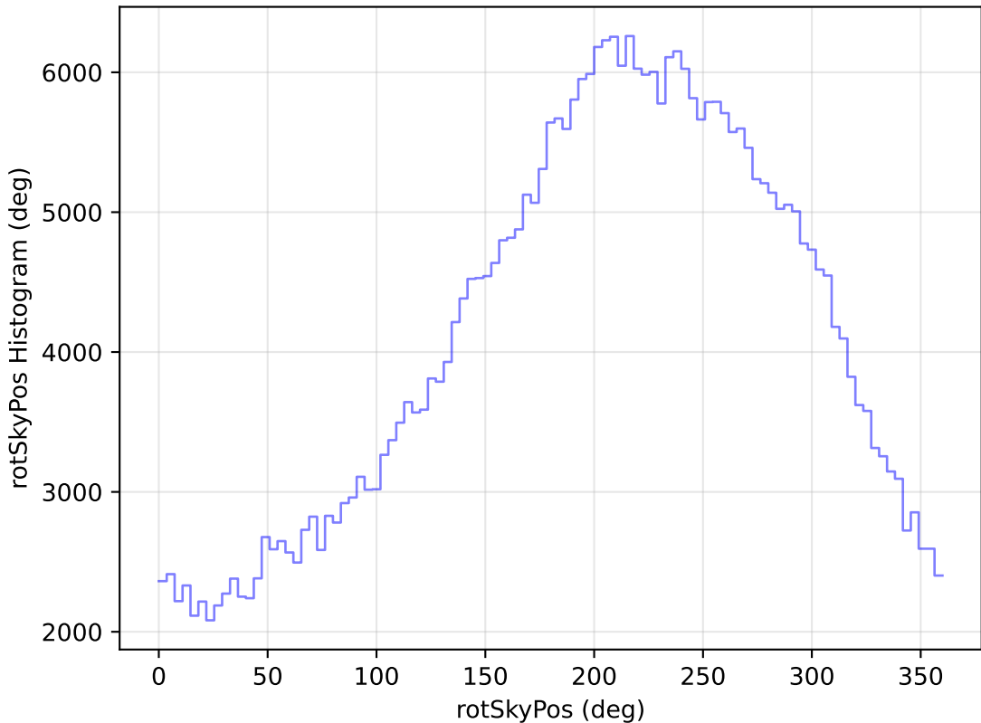
weather_cloudso35v3.4_10yrs All sky y band: rotSkyPos Histogram
