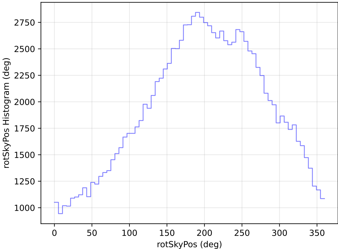
weather_cloudso35v3.4_10yrs All sky u band: rotSkyPos Histogram
