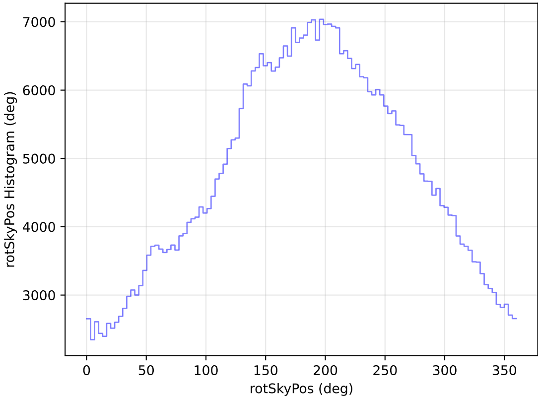
weather_cloudso35v3.4_10yrs All sky r band: rotSkyPos Histogram
