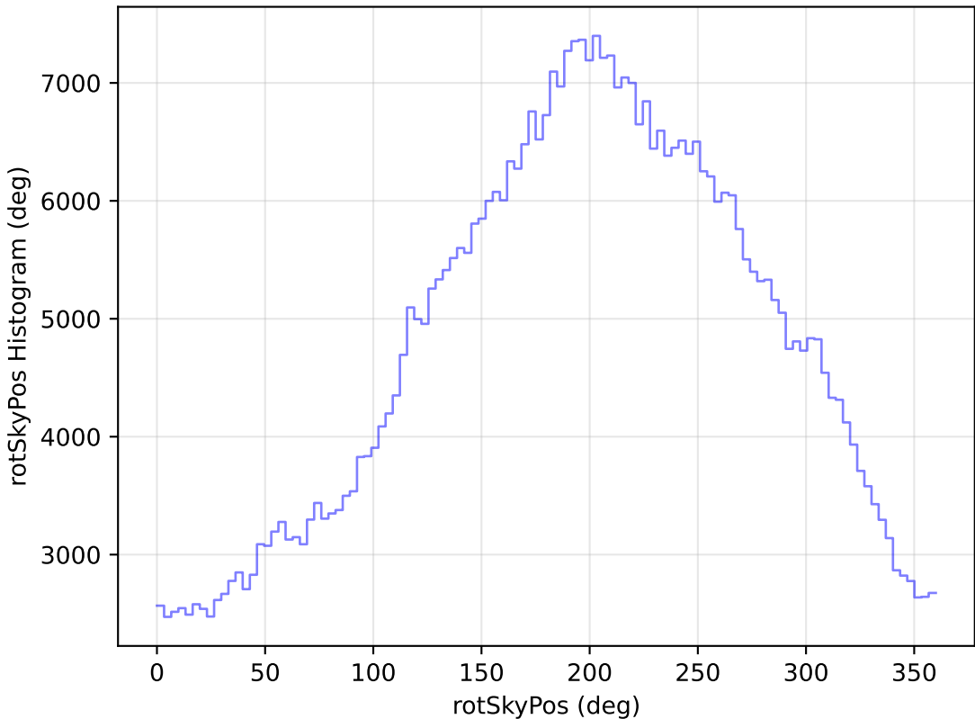
weather_cloudso35v3.4_10yrs All sky i band: rotSkyPos Histogram
