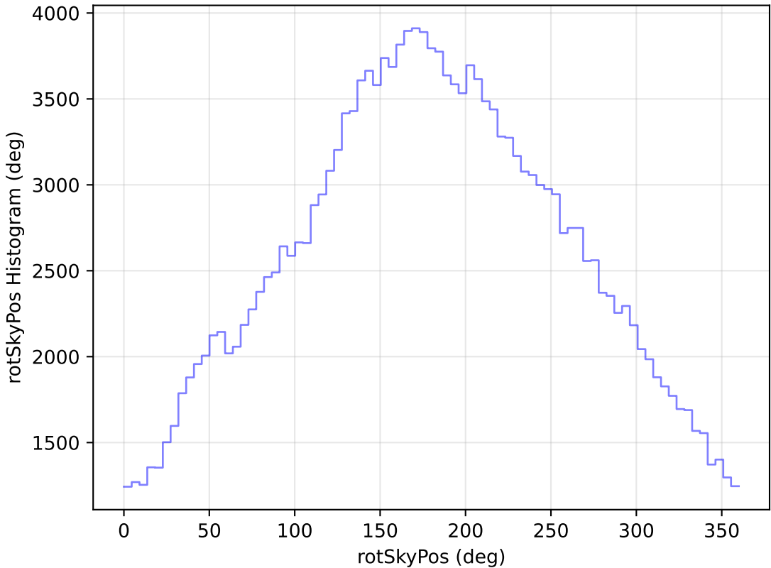
weather_cloudso35v3.4_10yrs All sky g band: rotSkyPos Histogram
