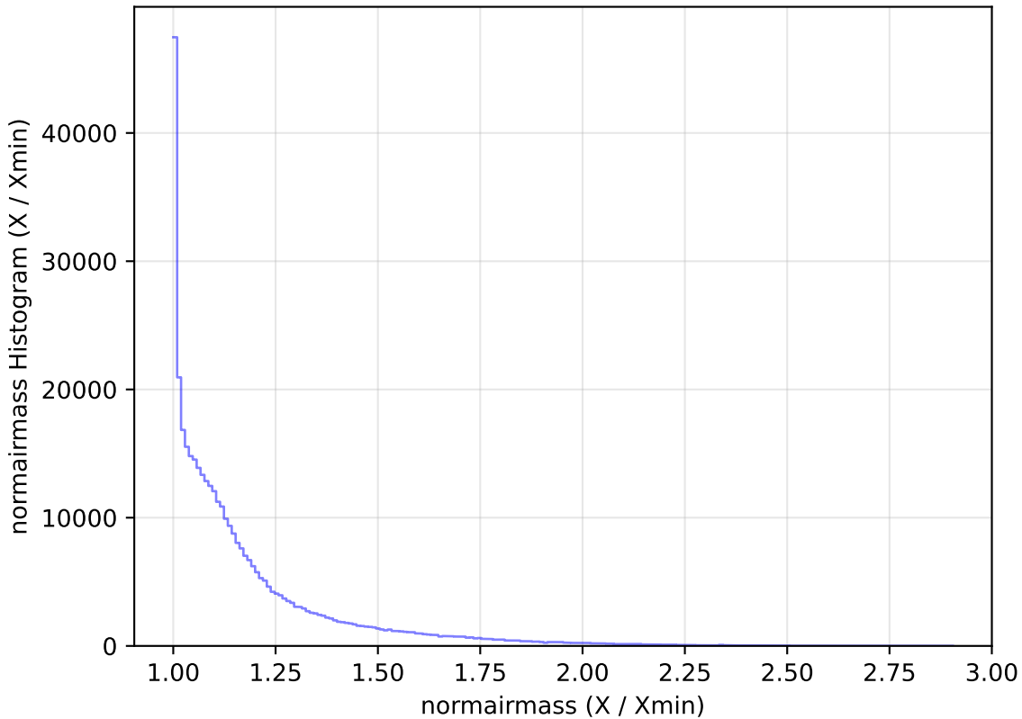
weather_cloudso35v3.4_10yrs WFD y band: normairmass Histogram
