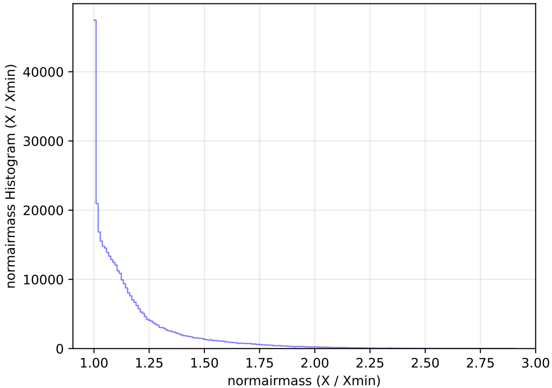
weather_cloudso35v3.4_10yrs All sky y band: normairmass Histogram
