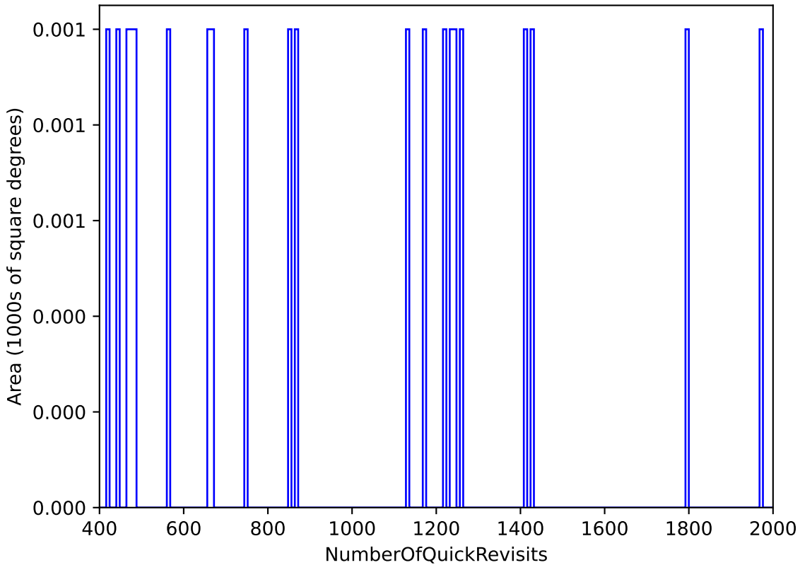
weather_cloudso35v3.4_10yrs All sky: NumberOfQuickRevisits
