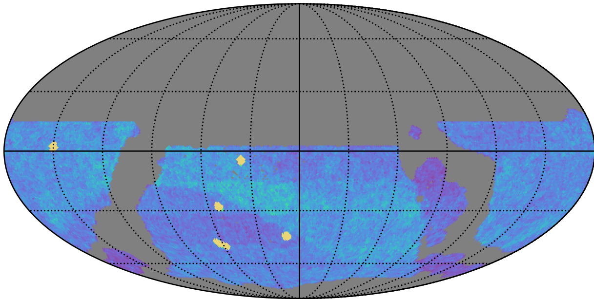
weather_cloudso35v3.4_10yrs WFD z band: NVisits
